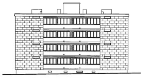
FACADE NORD
