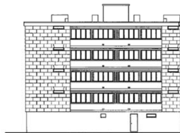
FACADE NORD
